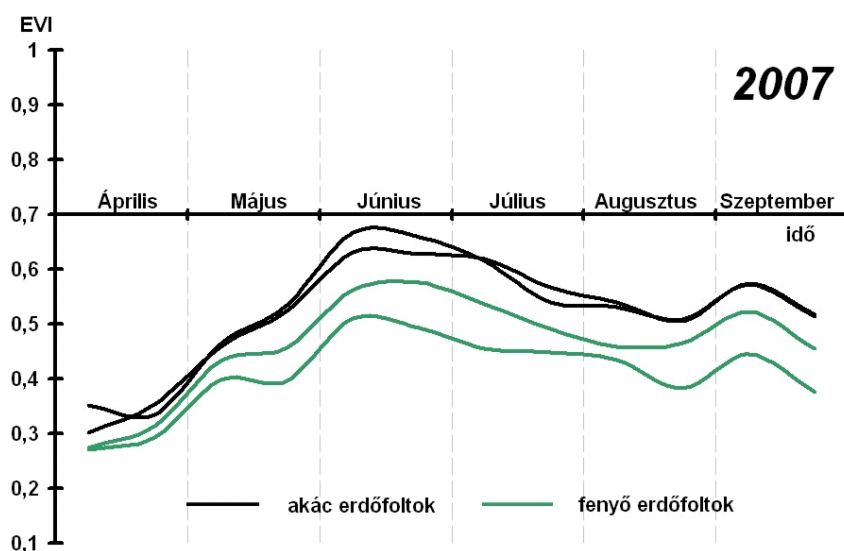
3. ábra. EVI vegetációs index átlagértékekből rajzolt vegetációs görbék illancsi fenyő és akác erdőfoltok esetén (2007).
