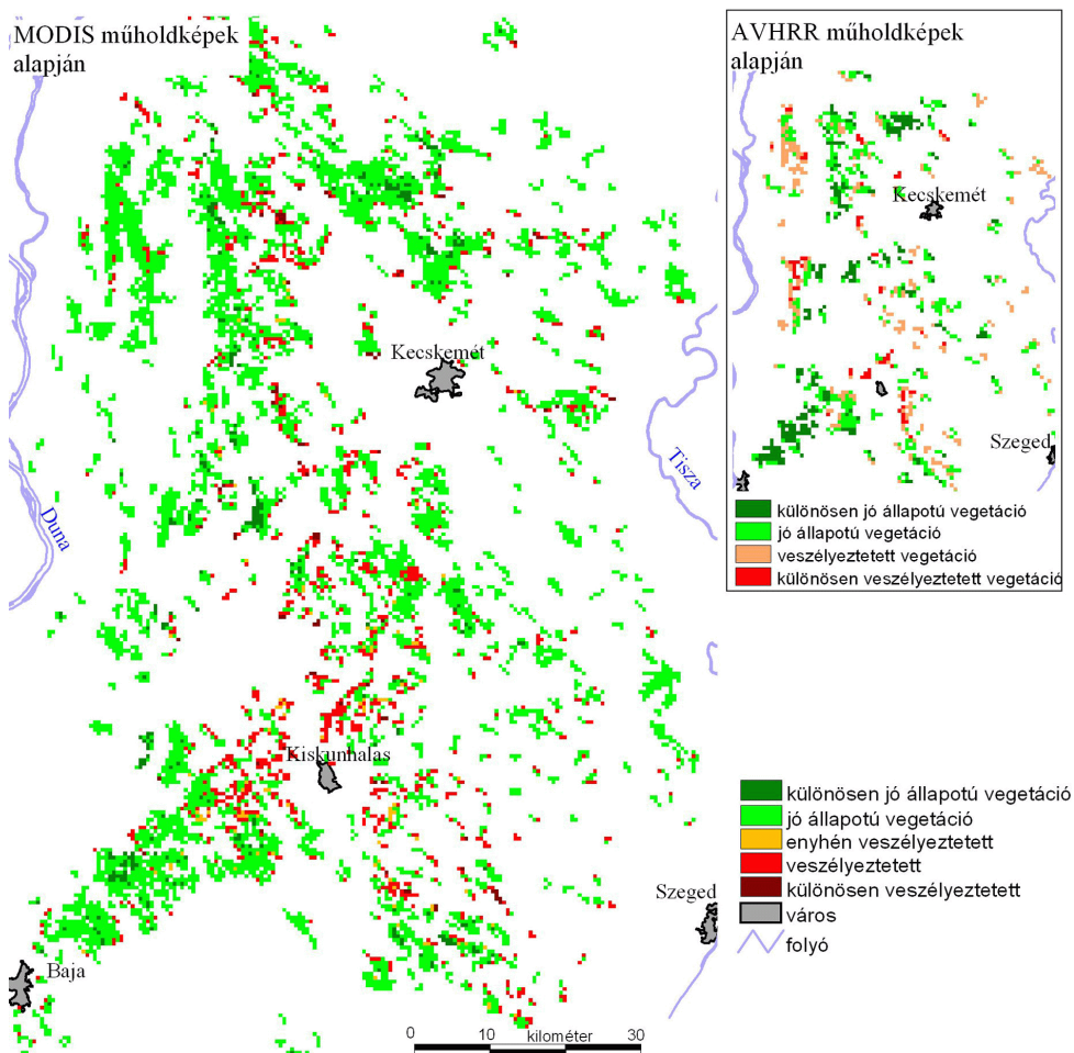
2. ábra. Klímaváltozás szempontjából veszélyeztetett területek lehatárolása az átlagtól való eltérés alapján.
